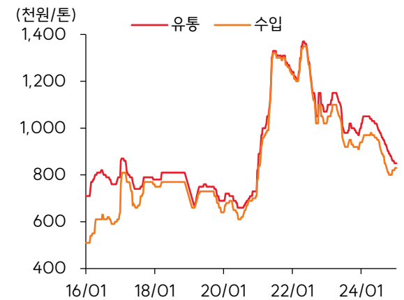
[철강] 국내 냉연 유통 및 수입 가격 추이
