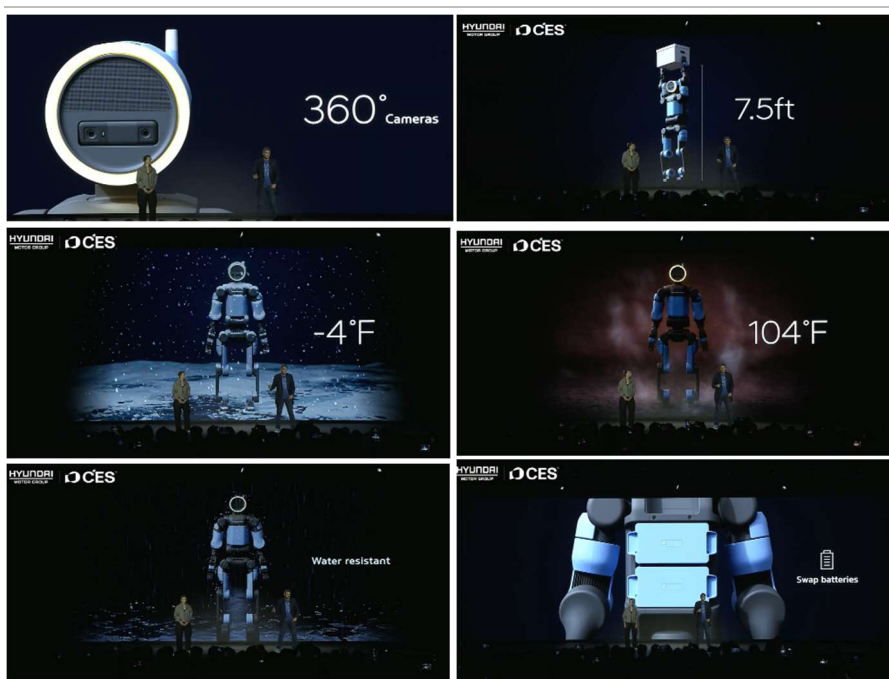
도표 4. Atlas 차세대 양산형 모델 주요 스펙
