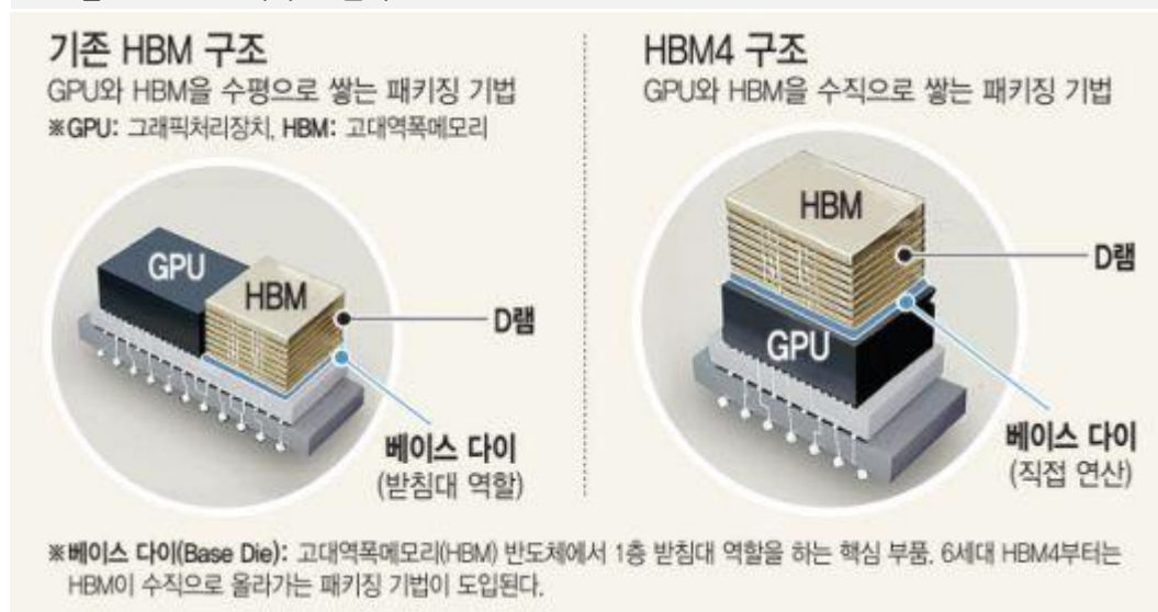
<그림10> HBM4의 구조 변화
