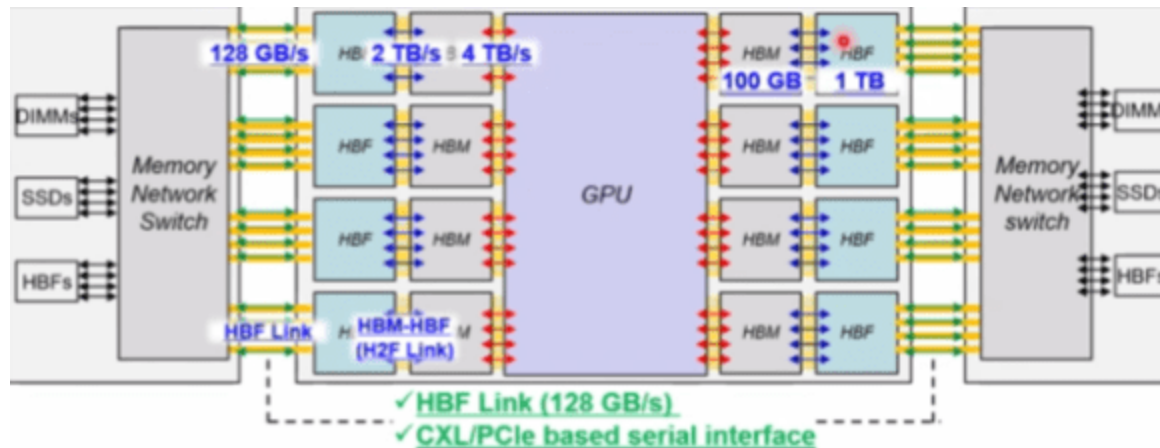
<그림21> AI 서버 내 HBM - HBF - Storage 구성도
