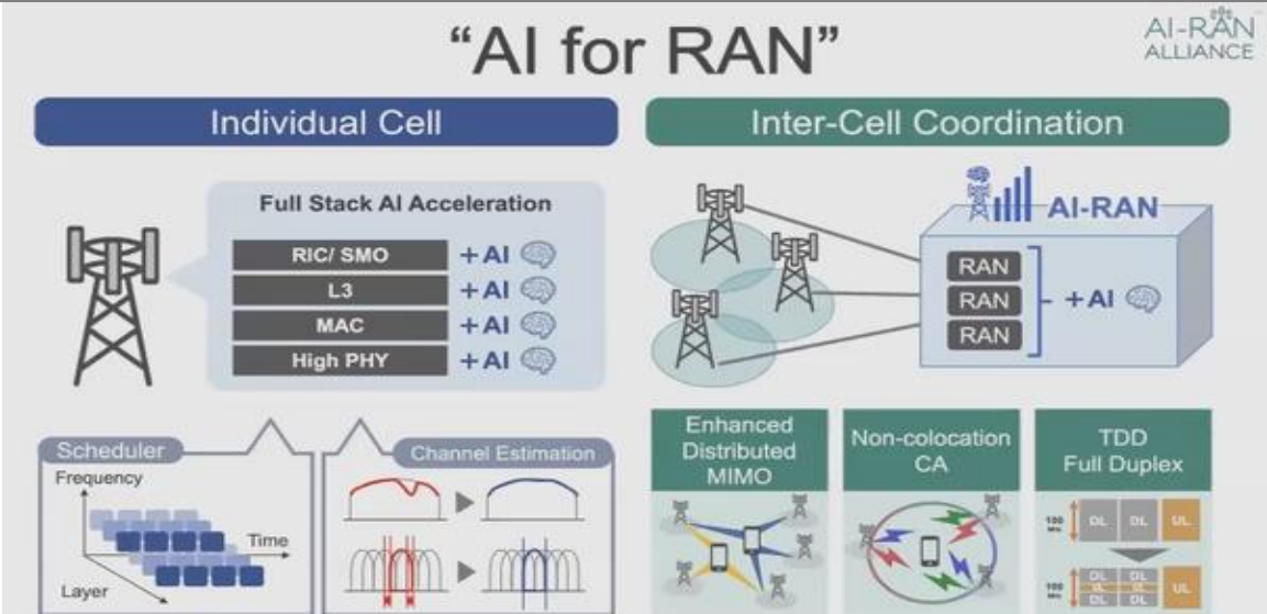
도표 1. AI 기지국 개념도
