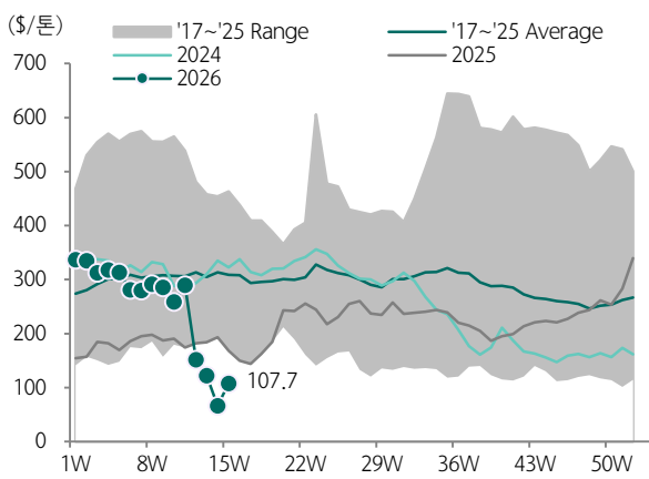
도표 127.PX 마진 추이
