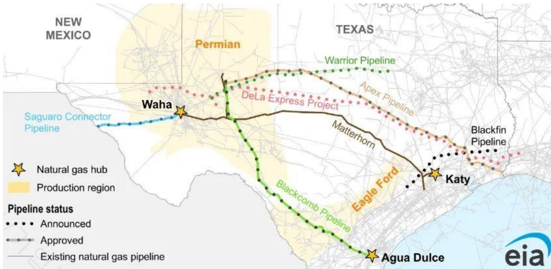
도표 1. Permian Waha에서 LNG 터미널까지 연결되는 주요 파이프라인 증설 현황
