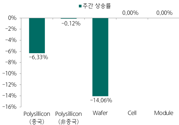
도표 26. 태양광 주요 체인별 제품가격 추이(PV Insight 기준)
