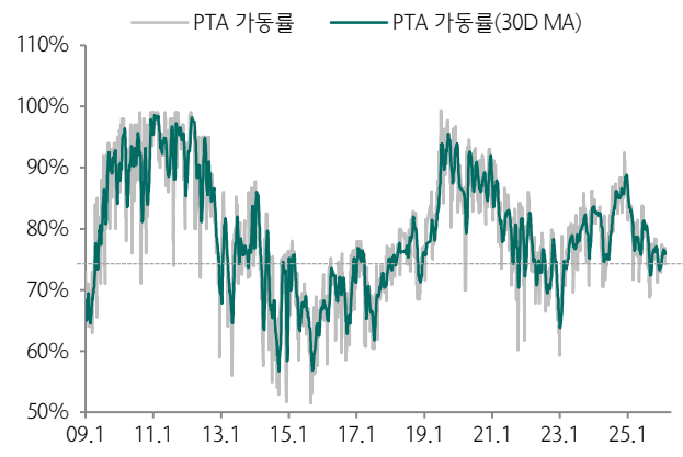
도표 97.중국 PTA 가동률 추이
