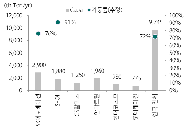
도표 54. 한국 PX 가동률 상향과 수출 확대 예상
