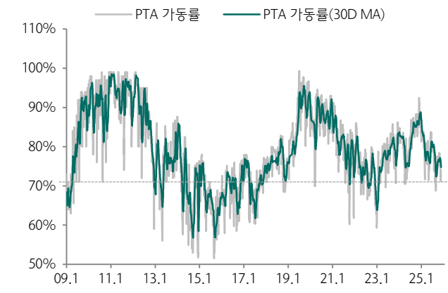
도표 98.중국 PTA 가동률 추이
