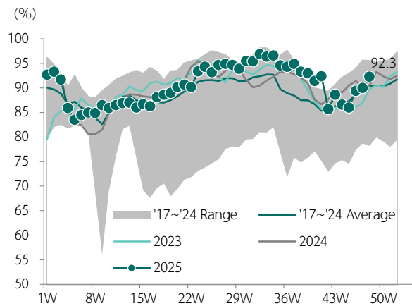
도표 149.미국 정유사 가동률 추이
