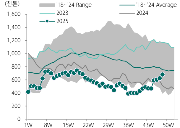
도표 88. 중국 동부 MEG 재고 추이
