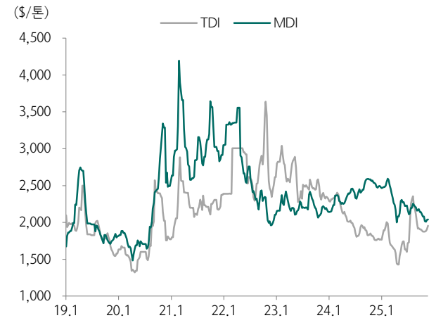
도표 138. MDI/TDI 가격 추이
