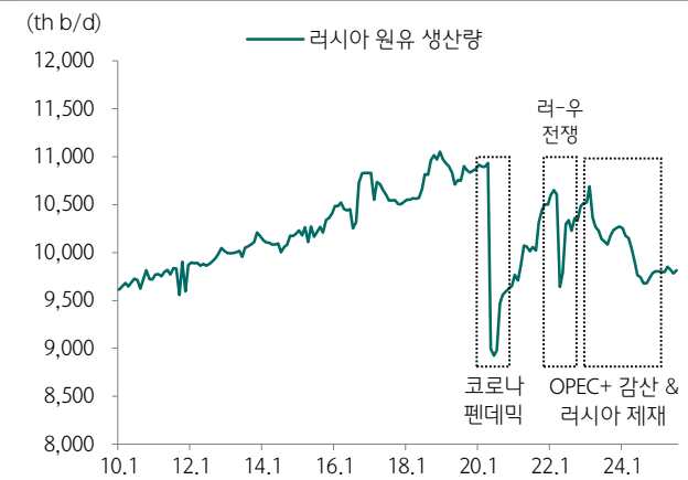
도표 4. 러시아 원유 생산량 추이
