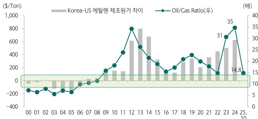
도표 1. Oil/Gas Ratio 15배 이하. 아시아 NCC와 미국 ECC의 경쟁력이 비슷해지기 시작하는 지점
