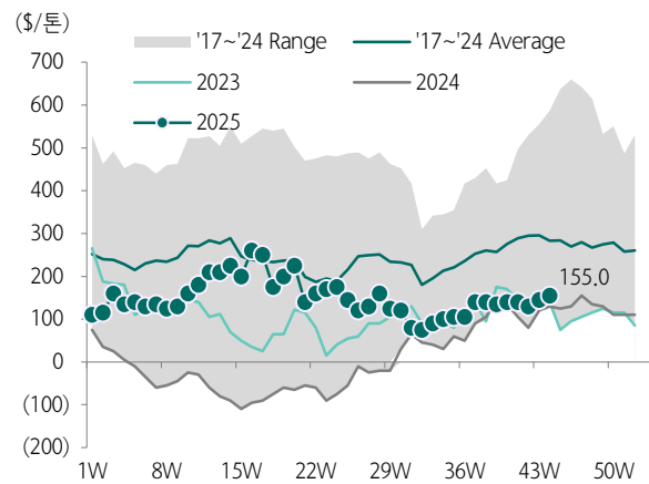
도표 129.페놀 마진 추이
