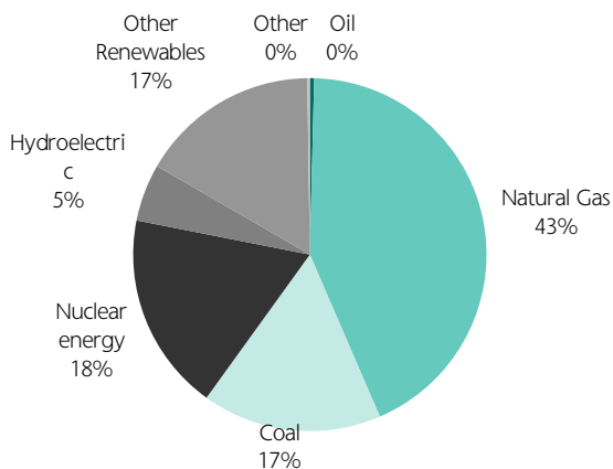
도표 119. 미국의 발전원별 발전 비중
