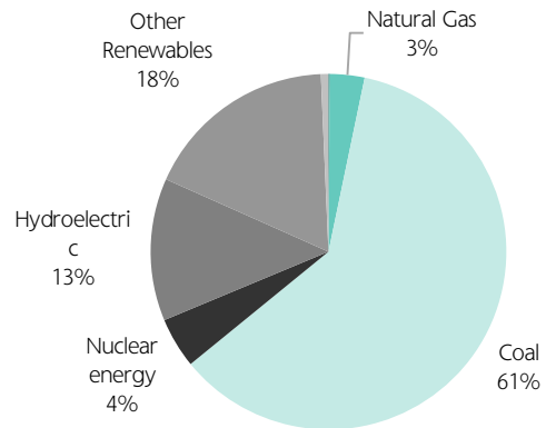
도표 125. 중국의 발전원별 발전 비중. 석탄이 압도적(61%)
