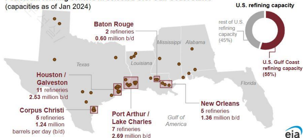
도표 74. 미국 정제설비의 55%가 Gulf Coast에 위치
