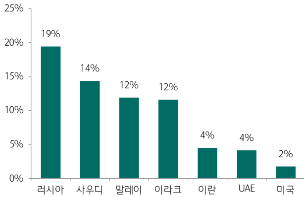
도표 107. 중국의 원유 수입 국가별 비중(이란산은 말레이 우회 수입)
