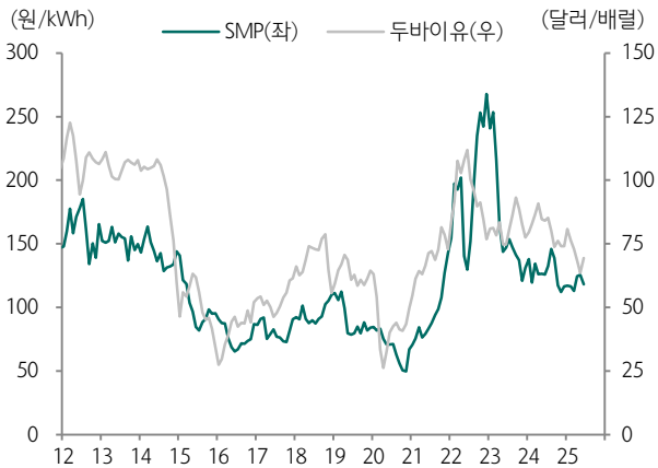
도표 3. SMP와 국제유가 추이 (6월 SMP YoY -6.3%)
