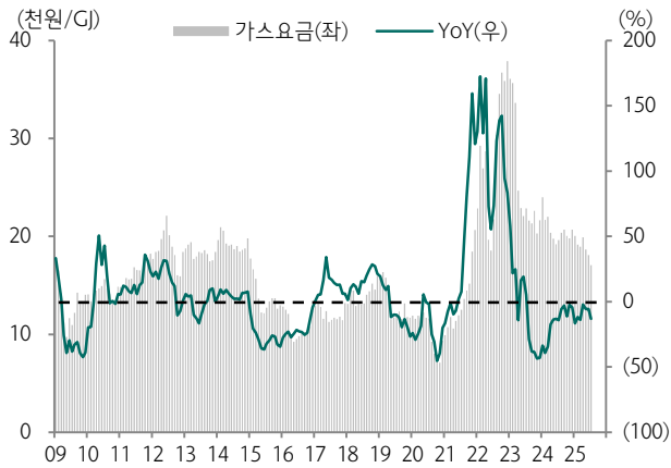
도표 1. 발전용 천연가스 가격 추이 (2025년 7월 YoY -13.1%)
