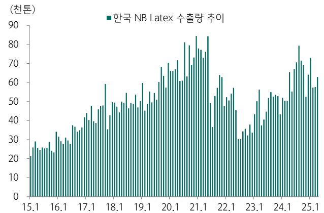
도표 67. 한국 NB Latex 수출량 4월부터 반등
