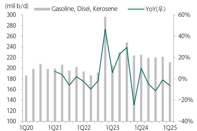
도표 50. 중국 PetroChina, 주요제품 생산량 YoY 감소세
