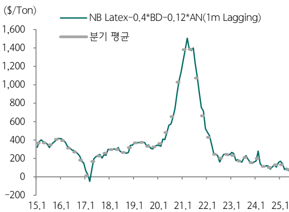
도표 206.NB Latex 마진 추이(1m lagging)
