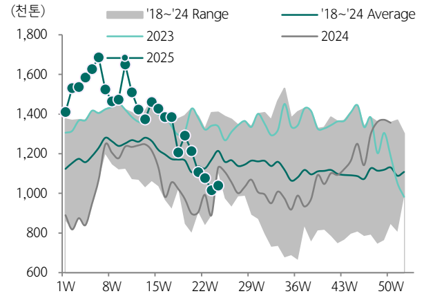
도표 251. 유럽 휘발유 재고
