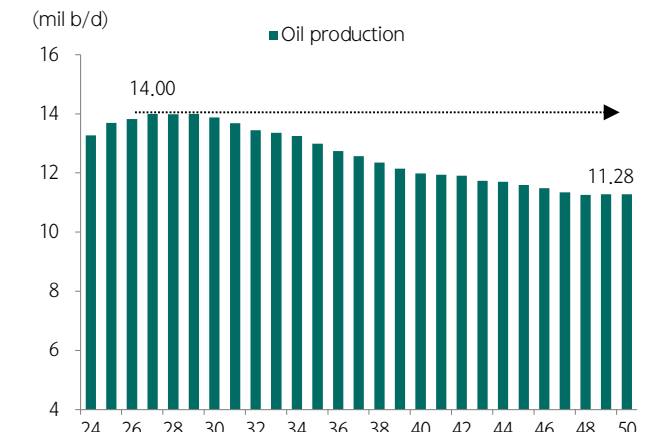
도표 69. EIA, 미국 원유 생산량 2027년 Peak를 예상
