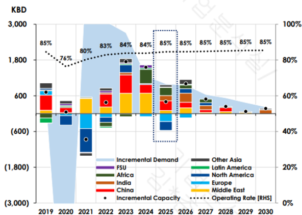
도표 58. 2025년 글로벌 CDU 증설 부담 완화 국면
