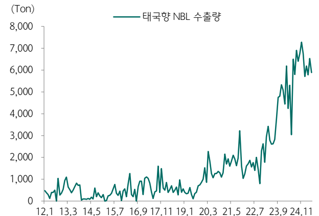
도표 209.NBL 태국향 수출량 추이
