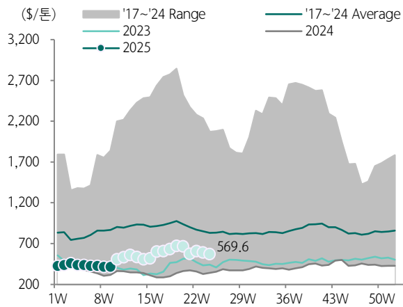
도표 210.BPA 마진 추이
