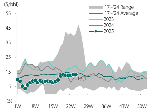
도표 235.휘발유 마진 추이
