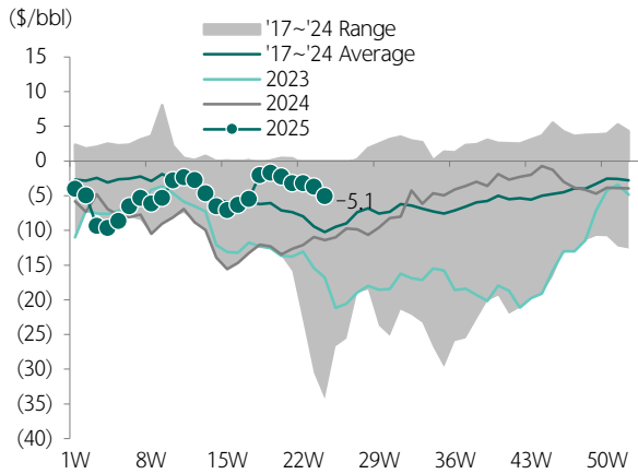
도표 238. 납사 마진 추이
