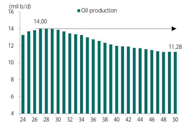
도표 56. EIA, 미국 원유 생산량 Peak 시점 2027년으로 전망
