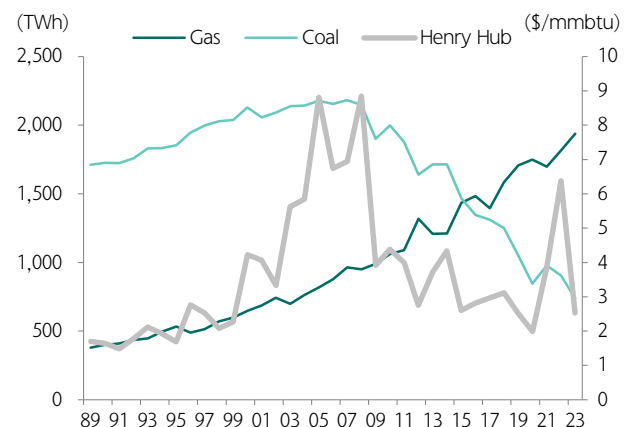
도표 75. 2000년 초, 발전수요 급증으로 HH 급등. ECC 경쟁력 하락
