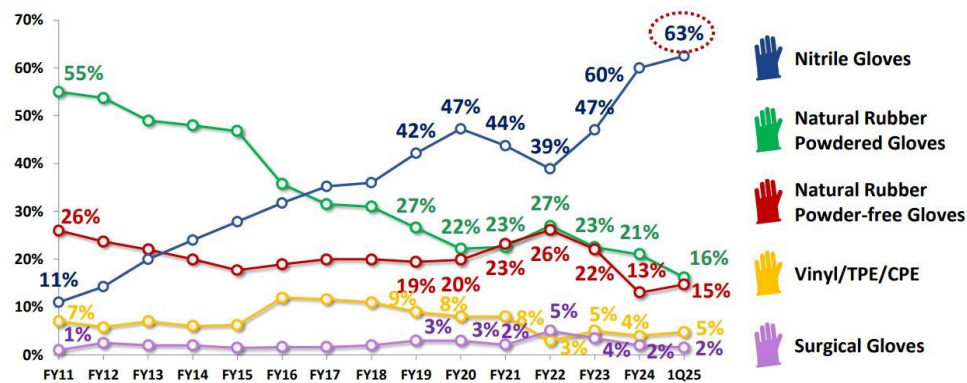
도표 114. Top Glove의 니트릴 장갑(NBL 사용) 생산 비중은 급증하고 있음
