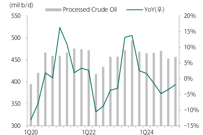
도표 43. 중국 Sinopec, 정제처리량 YoY 감소세
