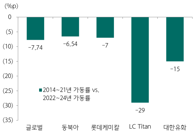
도표 103. 한국 NCC 업체들의 가동률은 동북아 대비 더 큰 폭의 조정
