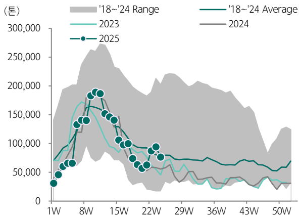
도표 180. 중국 동부 SM 재고 추이
