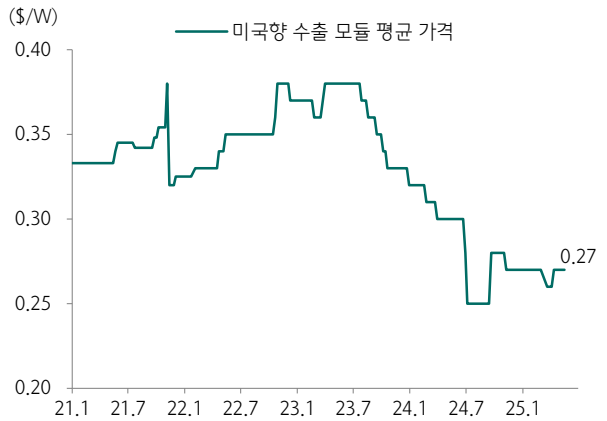
도표 28. 중국의 미국향 수출 모듈 평균가격 추이
