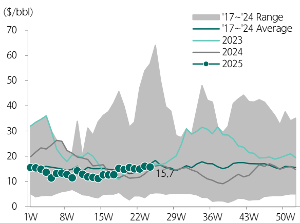
도표 236. 경유 마진 추이
