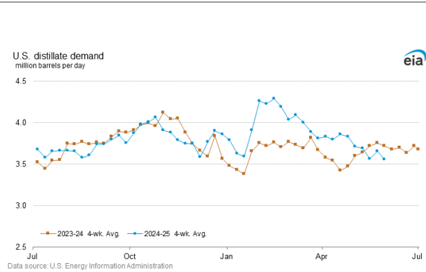
도표 234. 미국 등/경유 수요 추이
