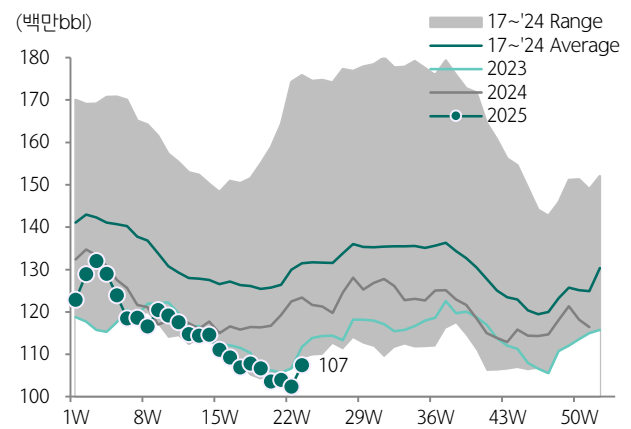
도표 233. 미국 등/경유 재고 추이
