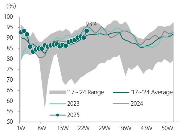
도표 230.미국 정유사 가동률 추이
