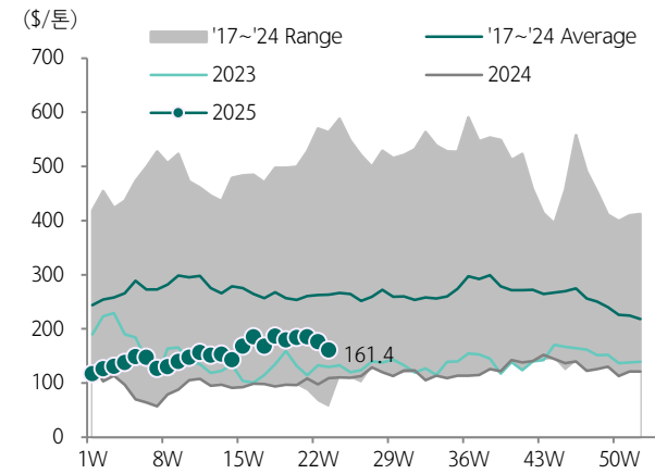
도표 206.SM 마진 추이
