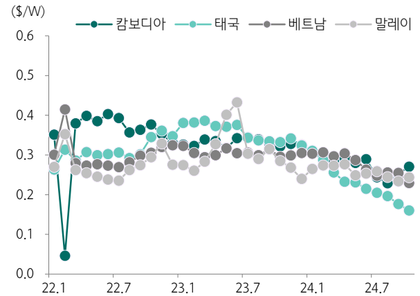
도표 132. 국가별 미국 태양광 모듈 수입 가격 추이
