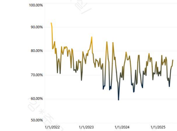
도표 211.중국 BPA 가동률 추이
