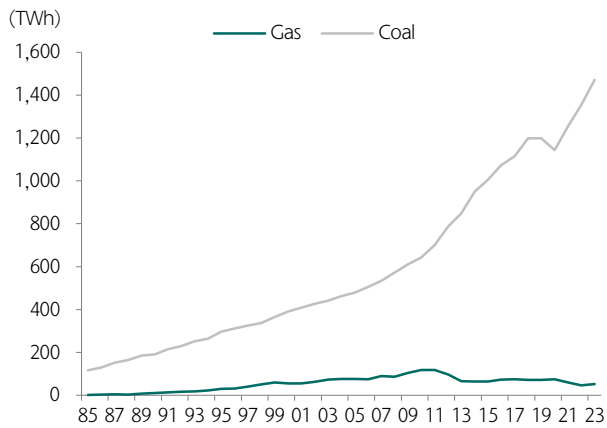
도표 164. 인도의 발전원별 발전량 비교(가스 vs. 석탄)
