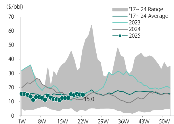
도표 228. 경유 마진 추이
