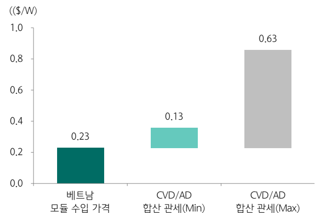
도표 122. AD/CVD 부과에 따른 베트남 모듈 가격 변화(M/S 23%)
