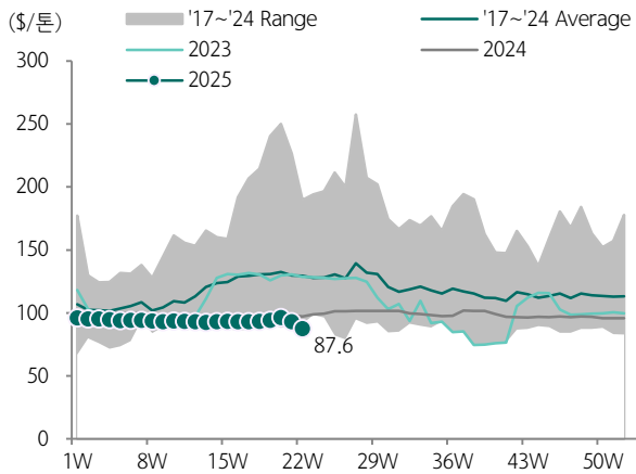
도표 190. PTA마진 추이(PX 차감 기준)
