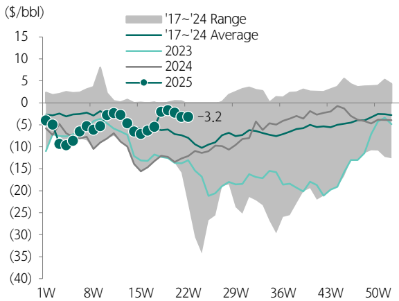
도표 230. 납사 마진 추이
