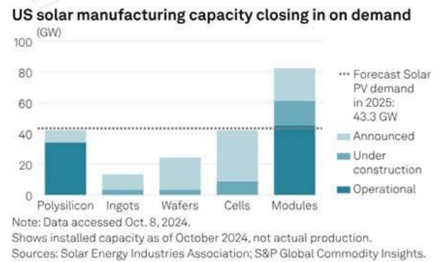
도표 118. 미국 모듈 Capa 약 40GW 대비 셀 Capa는 10GW 미만
