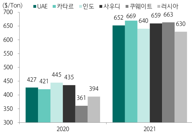
도표 140. 2020~21년 러시아 납사는 30~40$ 저렴하게 수입됨
