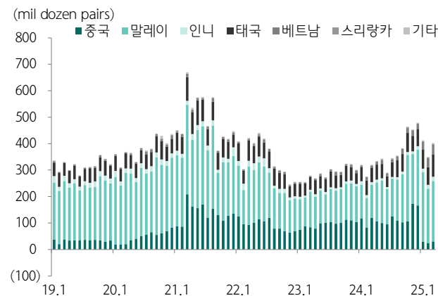
도표 39. 미국의 장갑 수입량 3월부터 회복세 시현 중
