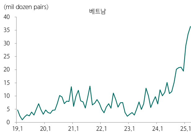
도표 45. 미국의 베트남산 장갑 수입량 급증 중
