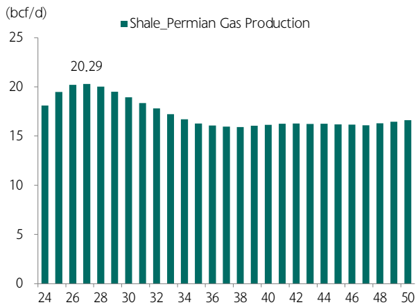
도표 38. Permian Basin의 Wet Gas 생산량은 2027년에 Peak
