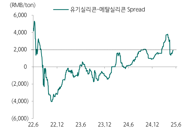
도표 214. 중국 메탈실리콘과 유기실리콘 스프레드
