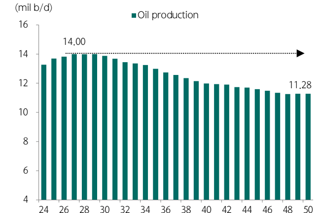
도표 37. EIA, 미국 원유 생산량 2027년 Peak를 예상
