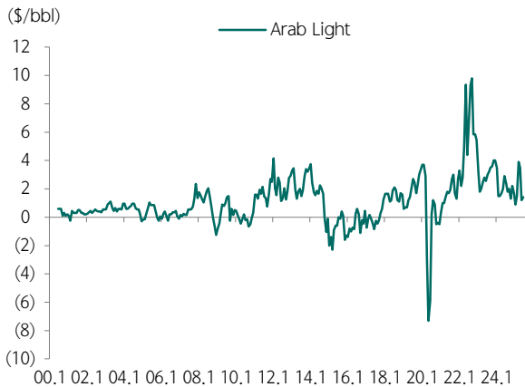
도표 40. 아시아 OSP 하향 안정화 예상
