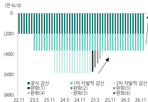
도표 36. 예상보다 가팔라진 OPEC+의 감산 완화 스케줄
