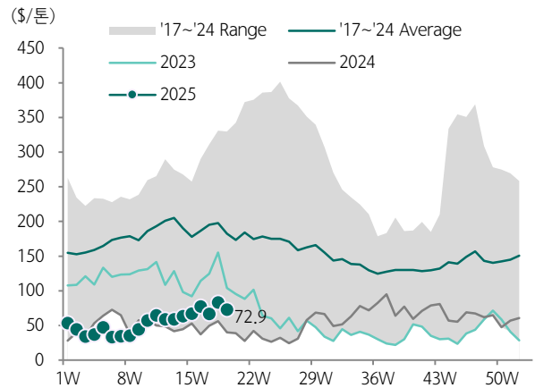
도표 188.PET마진 추이(MEG/PTA 차감 기준)
