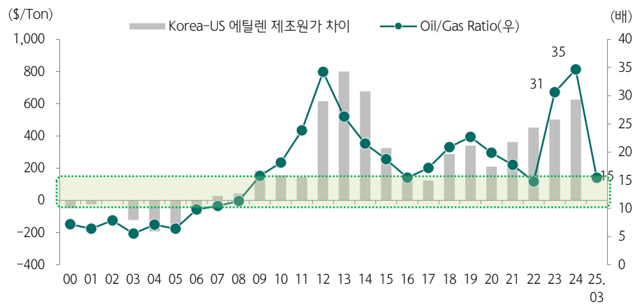
도표 48. Oil/Gas Ratio 15배로 아시아 NCC, 미국 ECC 간의 에틸렌 제조원가 차이가 유사해지는 구간에 진입
