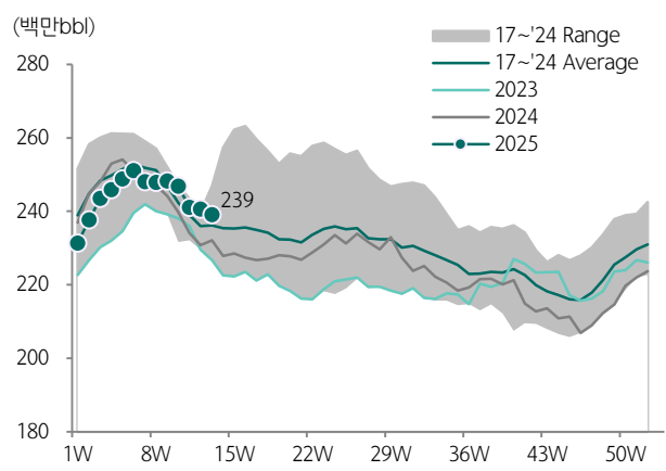
도표 216. 미국 휘발유 재고 추이
