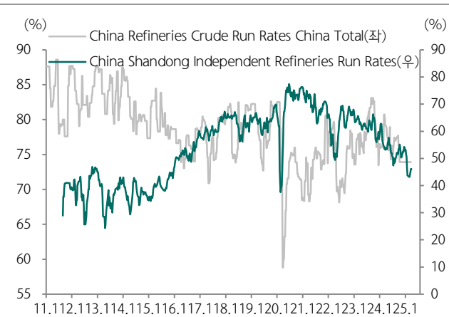
도표 221. 중국 국영/Teapot 가동률 추이
