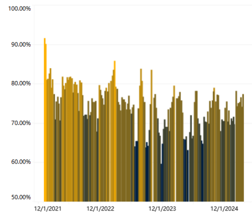
도표 196.중국 BPA 가동률 추이
