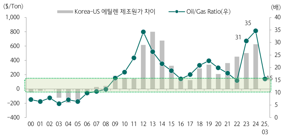
도표 42. Oil/Gas Ratio 15배로 아시아 NCC, 미국 ECC 간의 에틸렌 제조원가 차이가 유사해지는 구간에 진입
