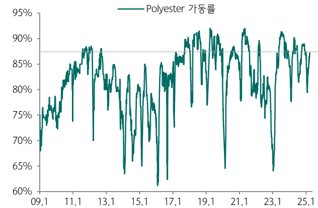
도표 163.중국 폴리에스터 가동률 추이
