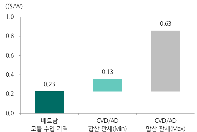
도표 103. AD/CVD 부과에 따른 베트남 모듈 가격 변화(M/S 23%)
