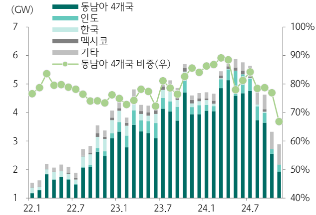
도표 78. 11월 미국 태양광 모듈 수입량 MoM-13% 감소
