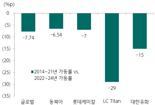
도표 56. 한국 NCC 업체들의 가동률은 동북아 대비 더 큰 폭의 조정
