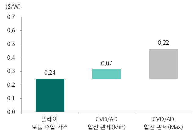
도표 99. AD/CVD 부과에 따른 말레이 모듈 가격 변화(M/S 11%)
