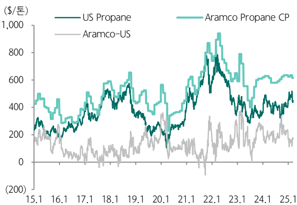
도표 145. 프로판 가격 추이
