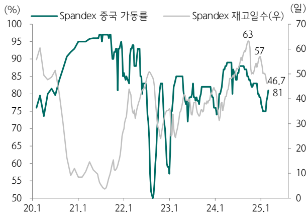
도표 189. 중국 Spandex 가동률과 재고일수
