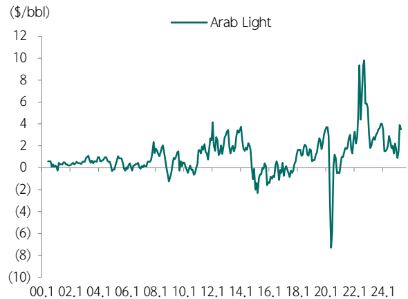
도표 210. 사우디 OSP 추이(Arab Light)
