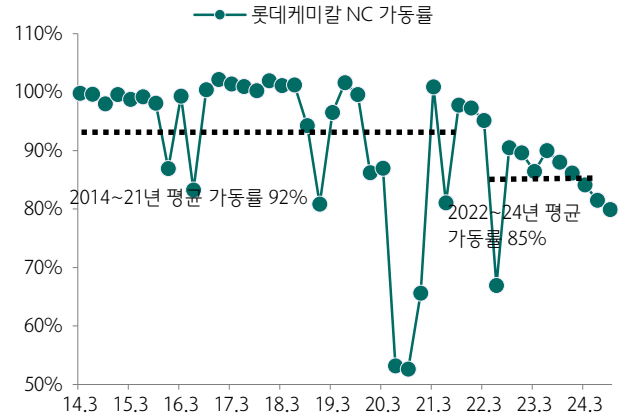
도표 50. 롯데케미칼 NCC 가동률 과거 대비 최근 -7%p
