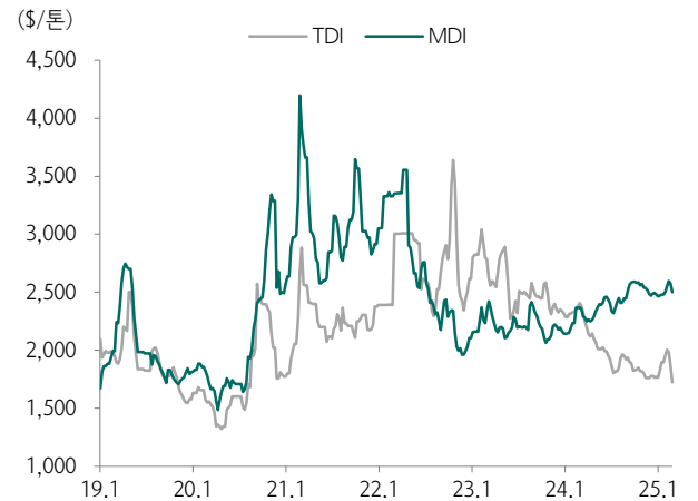
도표 192. MDI/TDI 가격 추이
