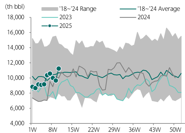
도표 211. 싱가포르 Mid Distillate 재고
