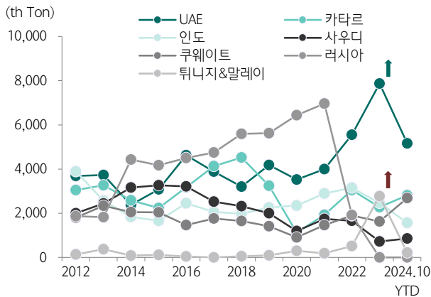
도표 106. 한국 납사 수입 국가별 물량. 2022년부터 러시아 납사 끊겨
