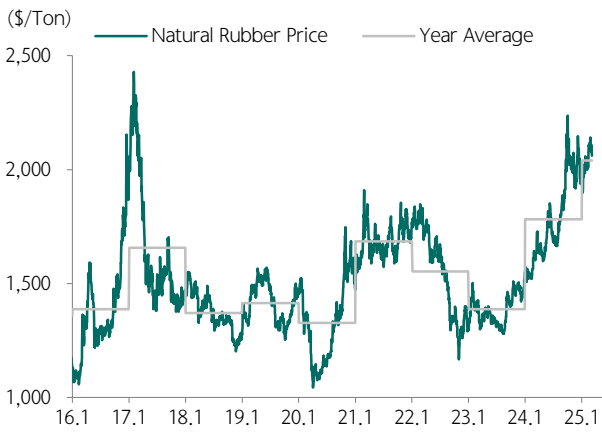
도표 163. 천연고무 가격 추이
