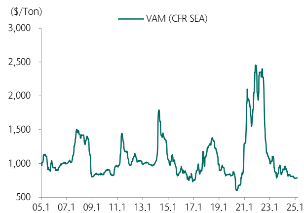
도표 183. VAM 가격 추이
