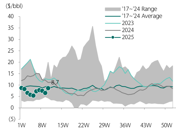
도표 197.정제마진 추이
