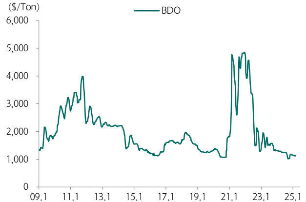
도표 190. Spandex 원재료 BDO 가격 추이
