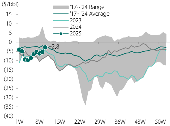
도표 201. 납사 마진 추이
