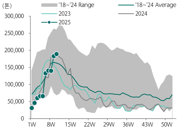
도표 143. 중국 동부 SM 재고 추이
