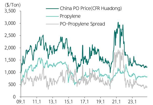
도표 194. 중국 PO 가격/마진 추이
