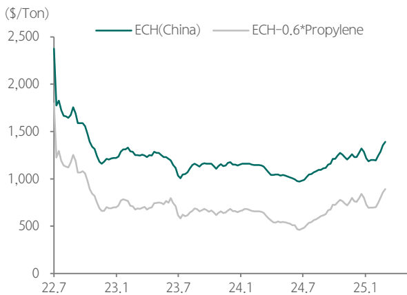
도표 6. 중국 ECH 가격/마진 추이
