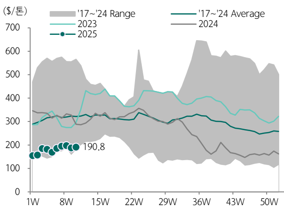
도표 159.PX 마진 추이
