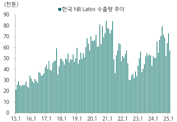
도표 168.한국 2월 NB Latex 수출물량 MoM -21.4%
