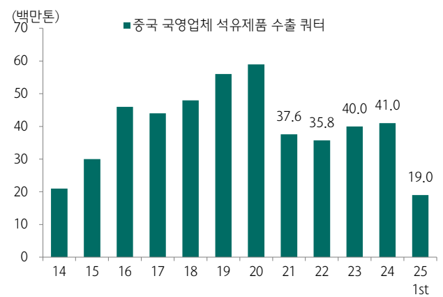
도표 11. 중국 석유제품 수출쿼터 추이
