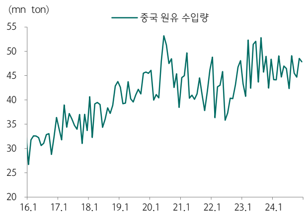
도표 9. 중국 원유 수입량 추이
