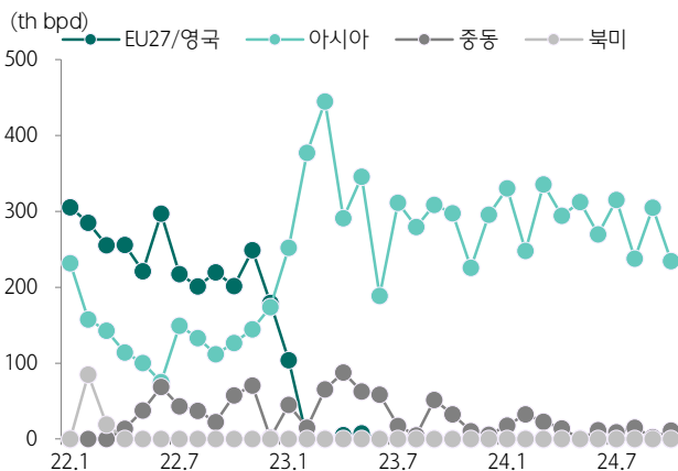
도표 108. 한국과 EU에서 러시아 납사는 사라져
