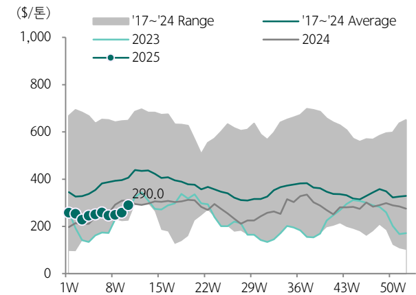
도표 153.에틸렌 마진 추이
