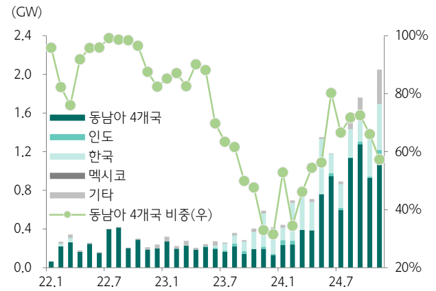
도표 86. 미국의 태양광 셀 수입량 급증 중
