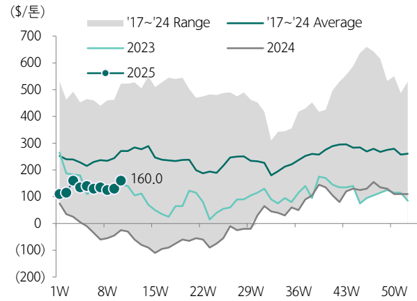
도표 174.페놀 마진 추이
