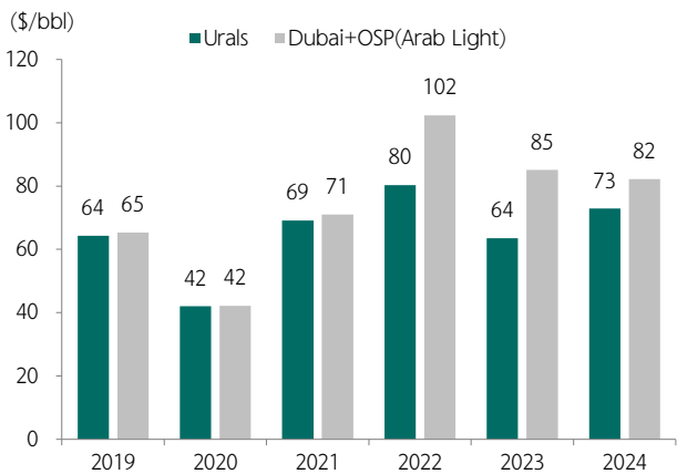
도표 102. 2022년부터 러시아 Urals, Dubai+OSP 대비 9~22$ 저렴
