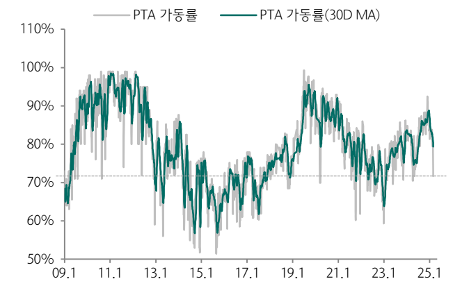
도표 152.중국 PTA 가동률 추이
