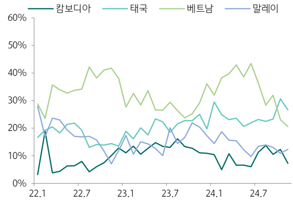
도표 75. 베트남으로부터의 태양광 모듈 수입량 크게 감소 중
