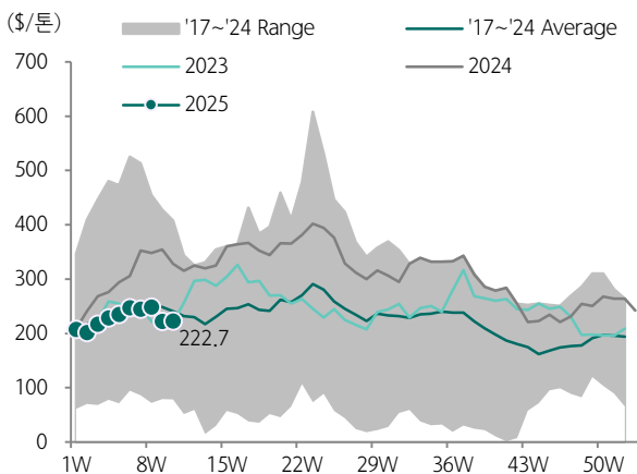
도표 177.벤젠 마진 추이
