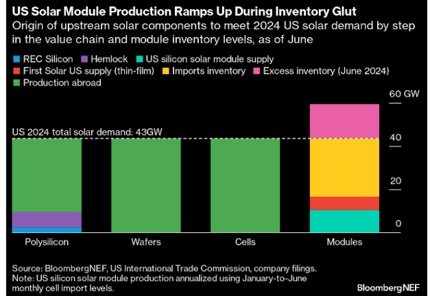
도표 123. 2024년 6월 기준 미국 태양광 모듈 재고는 43GW
