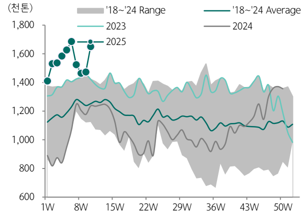
도표 214. 유럽 휘발유 재고
