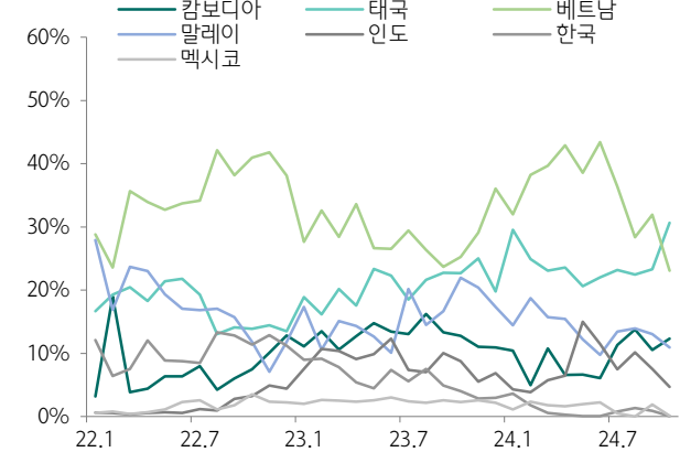
도표 99. 미국 태양광 모듈 수입 중 주요 국가의 M/S 변화 추이
