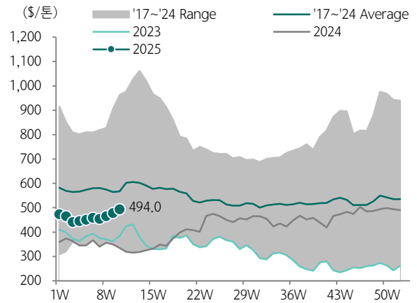
도표 156.LDPE 마진 추이
