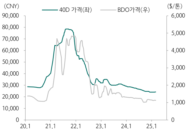
도표 191. 중국 스판덱스/BDO 가격 추이
