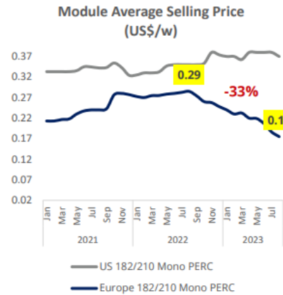
도표 25. 미국/유럽 모듈 평균 판매가격 비교
