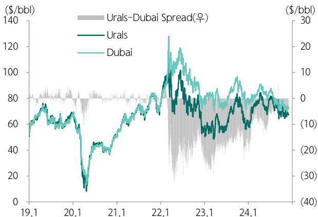
도표 104. Urals-Dubai 가격 추이
