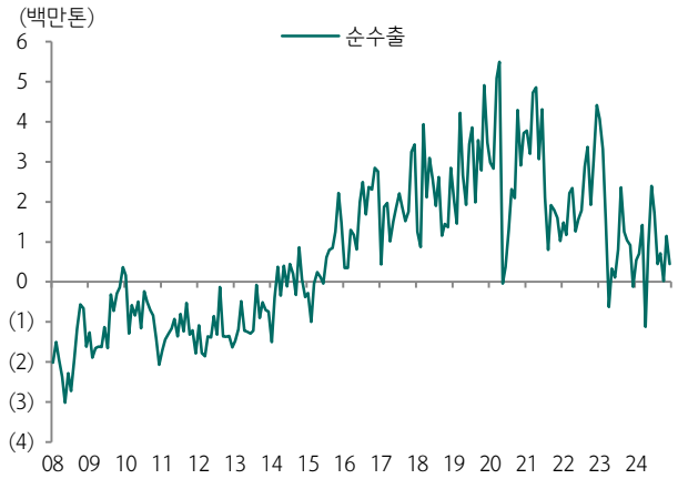
도표 208. 중국 12월 석유제품 순수출 MoM -61%
