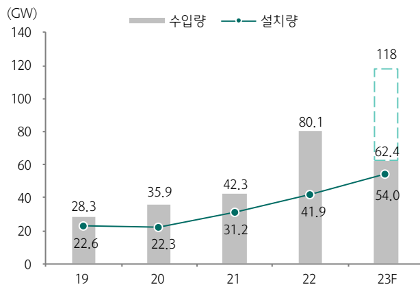
도표 24. 유럽 태양광 설치량과 모듈 수입량 비교
