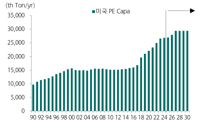
도표 38. 미국 대규모 PE 증설은 마무리 단계에 돌입
