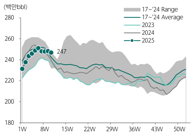
도표 204. 미국 휘발유 재고 추이
