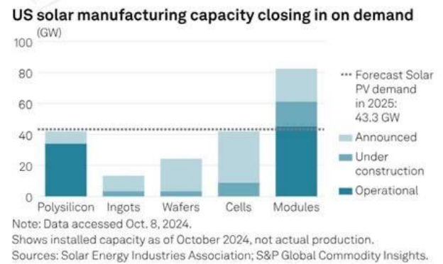
도표 85. 미국 모듈 Capa 약 40GW 대비 셀 Capa는 10GW 미만
