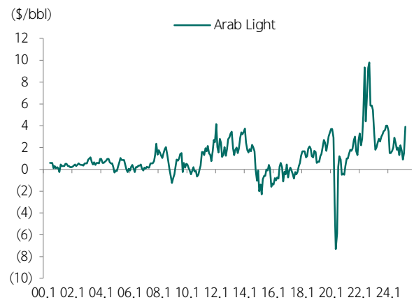
도표 197. 사우디 OSP 추이(Arab Light)
