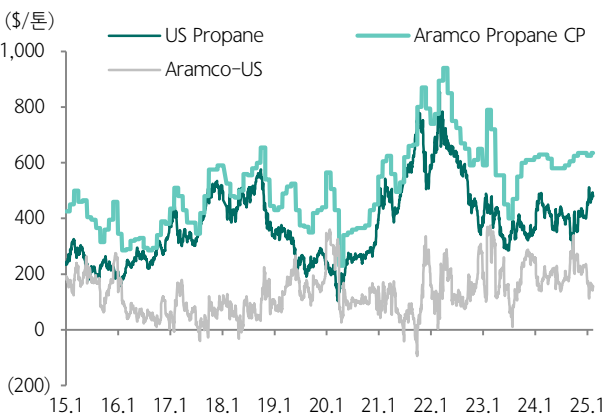
도표 128. 프로판 가격 추이
