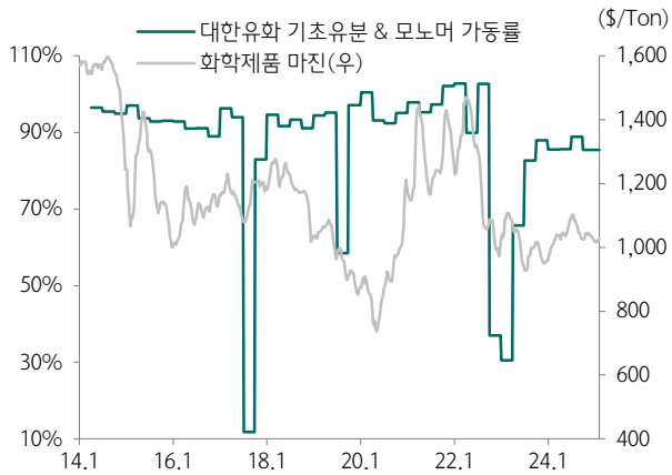
도표 11. 대한유화 NCC 가동률. 과거 업황 부진기 대비로도 낮아
