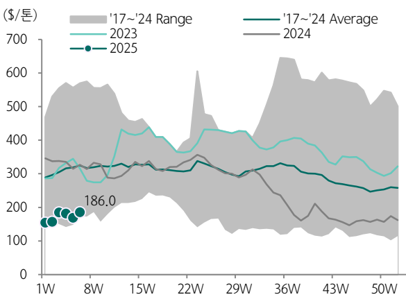
도표 170.PX 마진 추이
