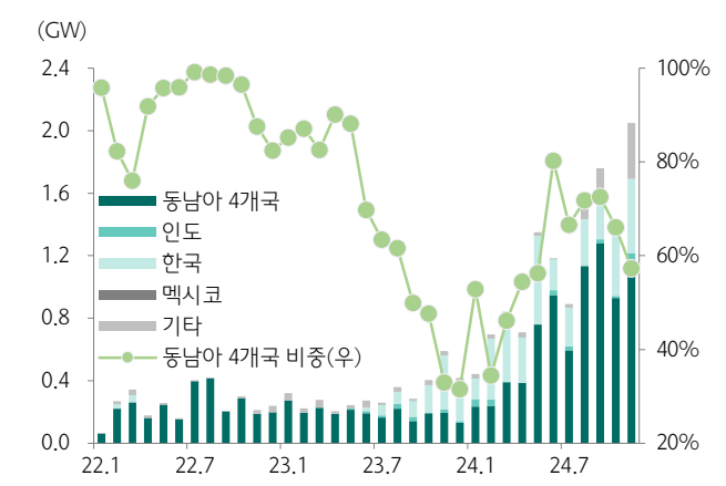
도표 52. 미국 태양광 셀 수입량 사상 최대
