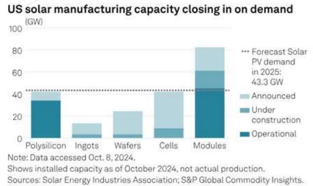
도표 63. 미국 모듈 Capa 약 40GW 대비 셀 Capa는 10GW 미만
