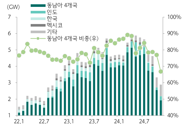
도표 49. 11월 미국 태양광 모듈 수입량 MoM-13% 감소
