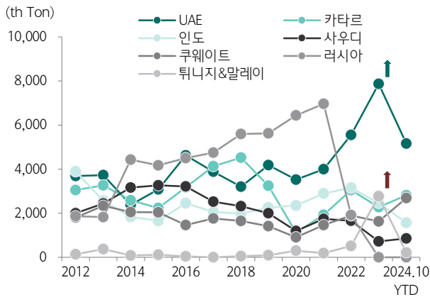
도표 81. 한국 납사 수입 국가별 물량. 2022년부터 러시아 납사 끊겨
