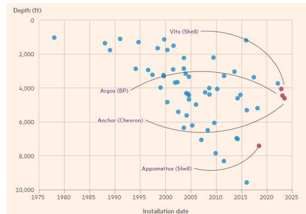
도표 100. 멕시코만(Gulf of Mexico)의 주요 심해 시추
