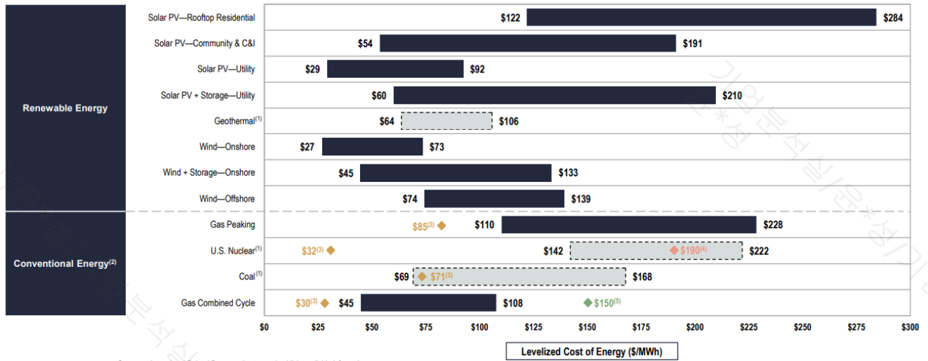
도표 130. 미국 발전원별 LCOE 비교
