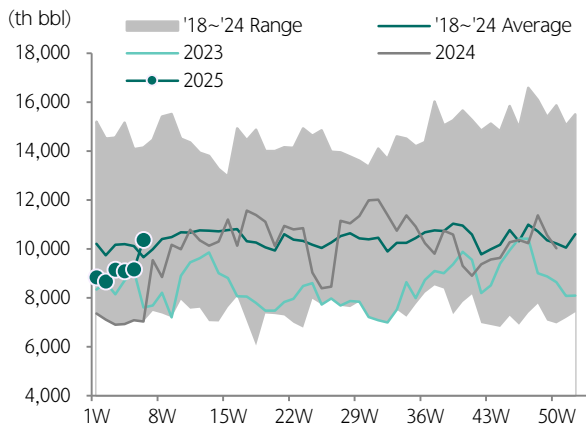
도표 223.싱가폴 Mid Distillate 재고
