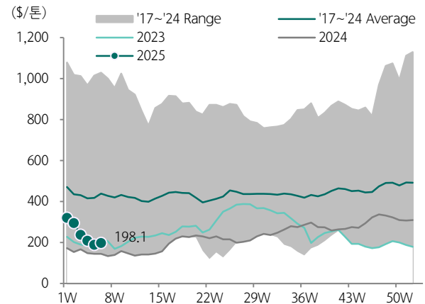
도표 177.ABS 마진 추이
