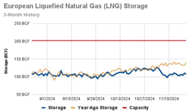
도표 119. EU 천연가스 재고는 YoY 20~30% 낮은 수준
