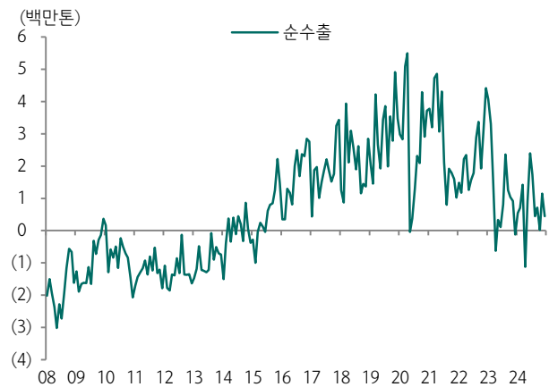
도표 220. 중국 12월 석유제품 순수출 MoM -61%
