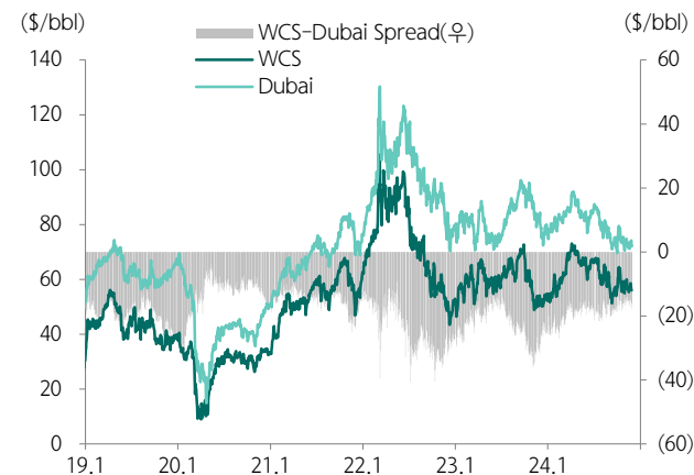
도표 112. Dubai와 WCS 간의 가격 차이는 약 16$/bbl 수준
