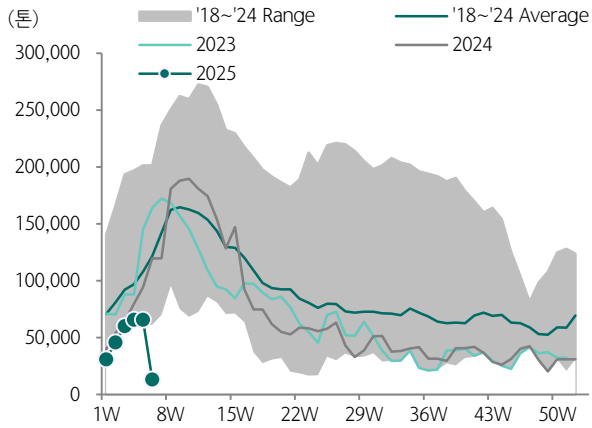
도표 154. 중국 동부 SM 재고 추이
