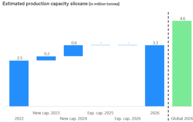
도표 140. 중국 실록산 생산 Capa는 2024년 증설 이후 2025~26년 전무한 구간에 진입
