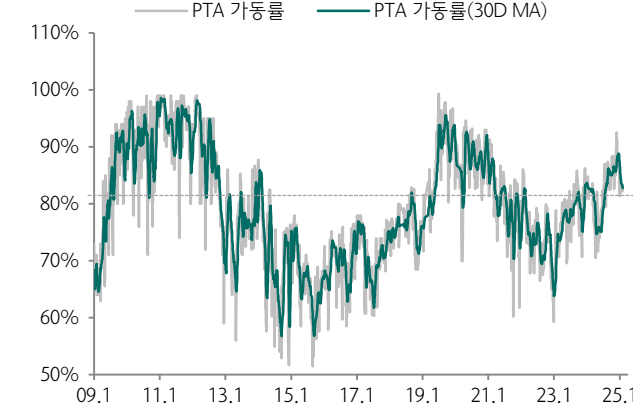
도표 163.중국 PTA 가동률 추이
