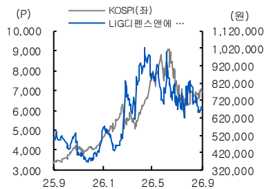
LIG디펜스엔에어로스페이스 상대주가 (%)
