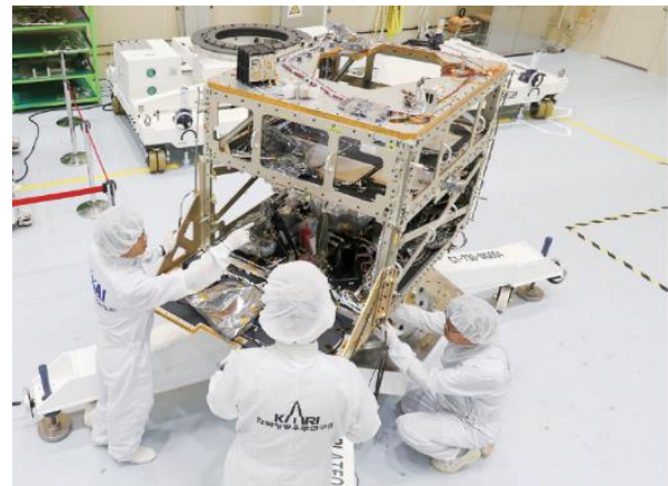
그림 164. 조립 중인 차세대중형위성
