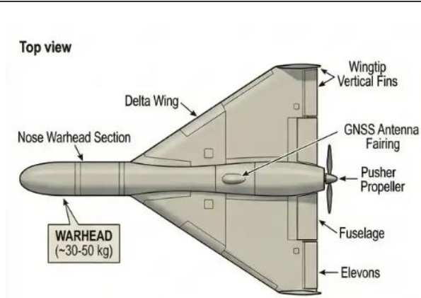
그림 179. 러시아-우크라이나 전쟁에서 사용된 Shahed-131
