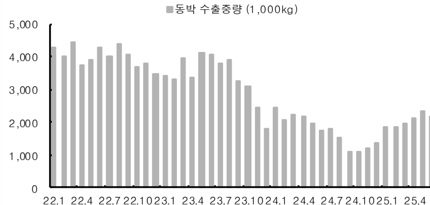
동박 수출증량
