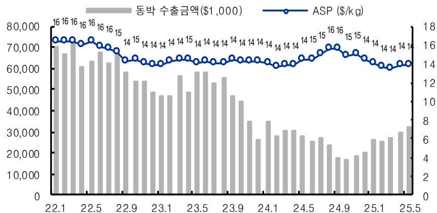
동박 수출금액
