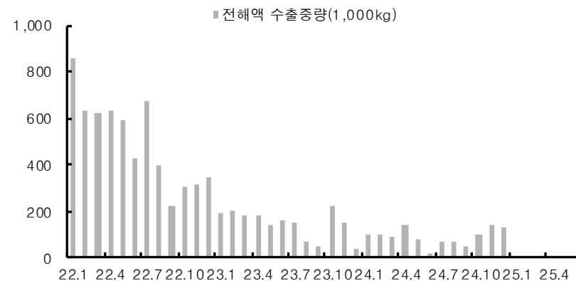
전해액 수출증량
