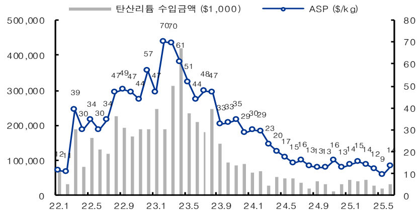
탄산리튬 수입금액
