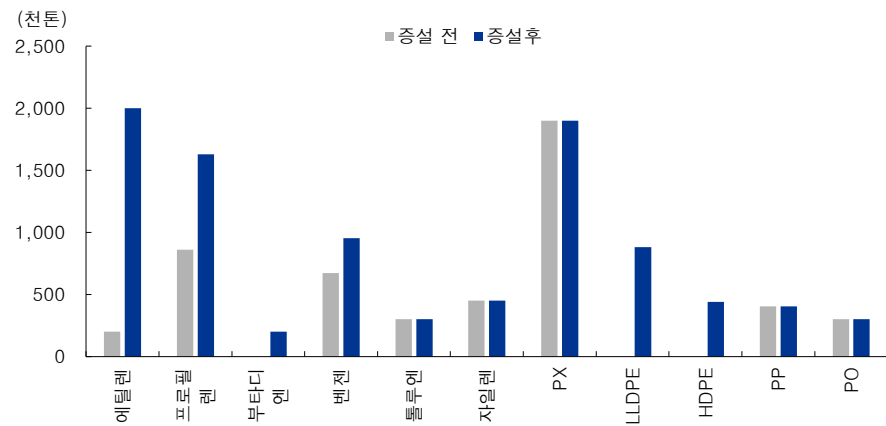
그림 39. S-Oil 사한 프로젝트 증설 전/후 화학 제품 생산능력 비교
