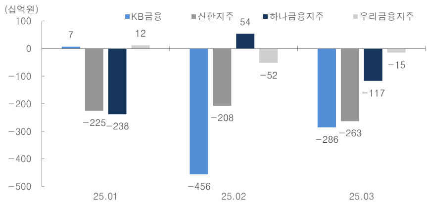
그림 1. 커버리지 2025년 외국인 순매수대금 추이
