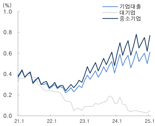
그림 3. 원화대출 연체율 추이_기업
