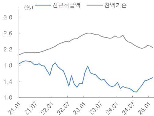
그림 4. 예금은행 가중평균금리 금리차
