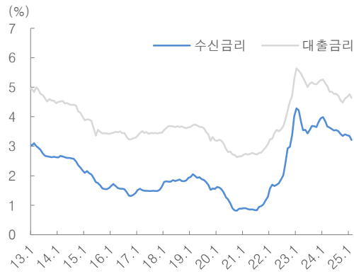
그림 5. 예금은행 가중평균금리_신규 취급액 기준
