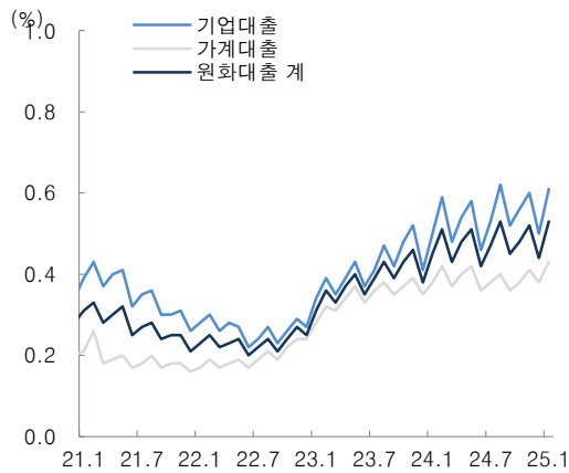
그림 2. 원화대출 연체율 추이_전체
