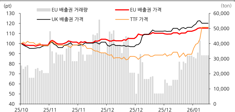
[그림1] EU 탄소배출권 및 TTF 가스 상대가격 추이
