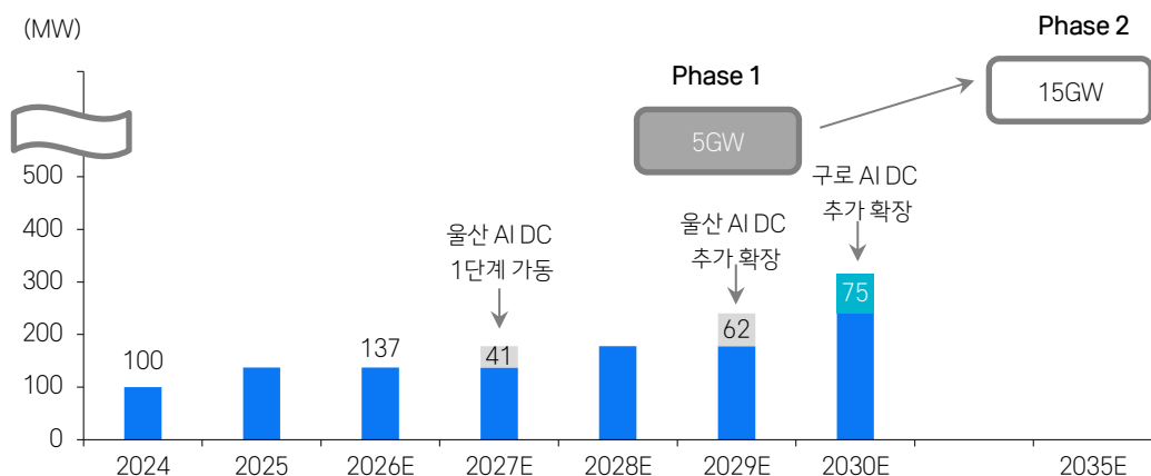
그림 6. SK텔레콤의 데이터센터 용량 및 확장 계획
