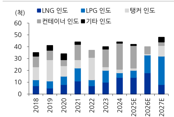
도표 3. 선박 딜리버리 스케줄
