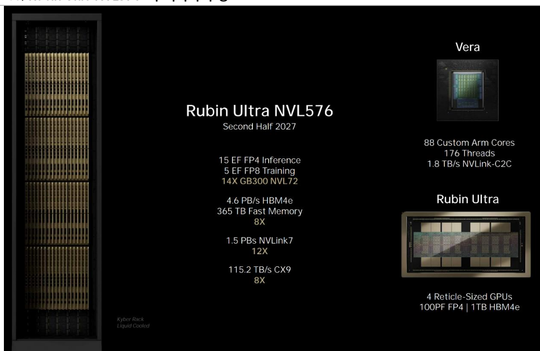
도표 16. Rubin Ultra NVL576 랙 서버의 구성
