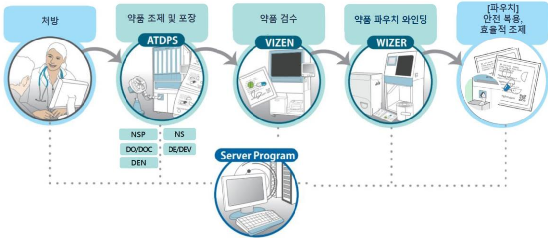
그림8. 제이브이엠 조제 자동화 업무 프로세스
