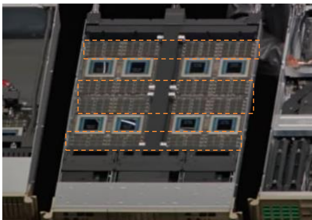
그림10. Vera CPU 전용 트레이에 빼곡히 탑재된 SOC&MM 모듈
