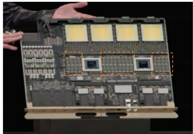
그림11. VR Ultra 컴퓨트 트레이에 탑재된 SOC&MM 모듈
