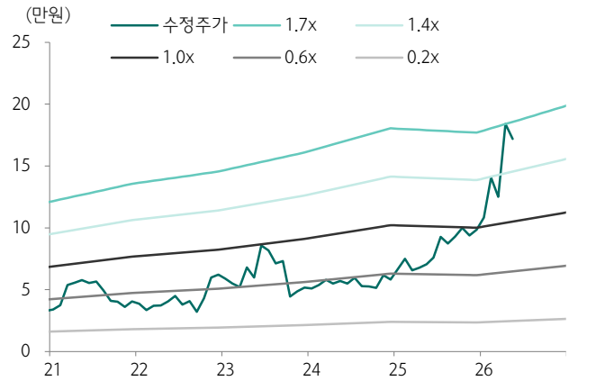
도표 3. HD건설기계 12M Fwd PBR
