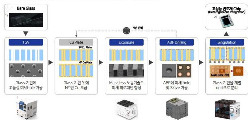
도표 4. 글라스 기판 생산공정
