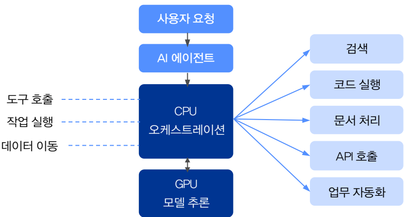
그림 3. 에이전틱 AI 워크로드: 추론·계산은 GPU, 나머지 실행 전반은 CPU가 담당
