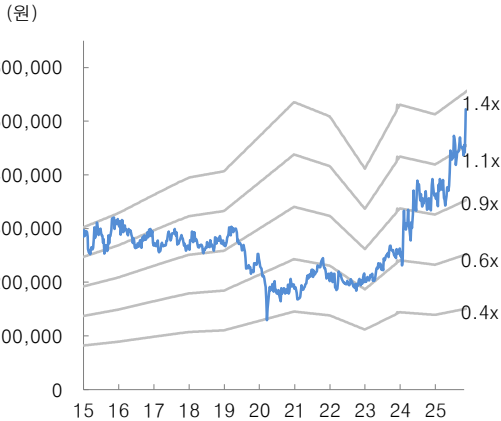
그림 8. 삼성화재 PBR 밴드
