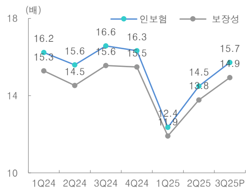
그림 3. 삼성화재 CSM 배수 추이
