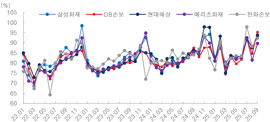
그림 5. 주요 손해보험사 자동차보험 손해율 추이
