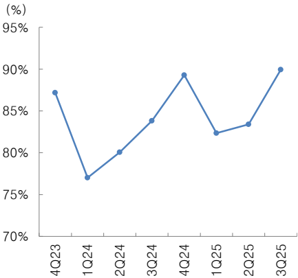
그림 9. 삼성화재 자동차보험 손해율 추이
