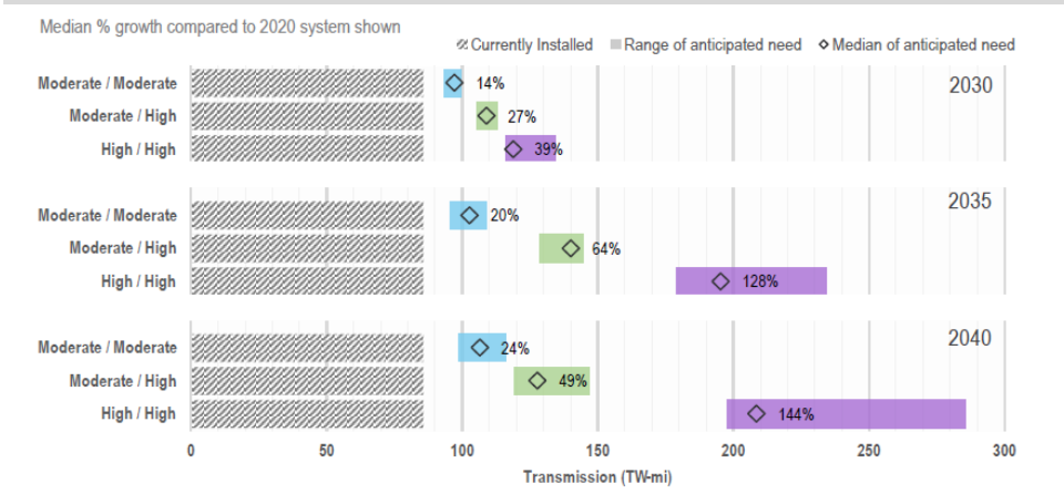
그림 8. 미국의 2035/2040년까지 지역(주) 내 송전용량 요구치 전망
