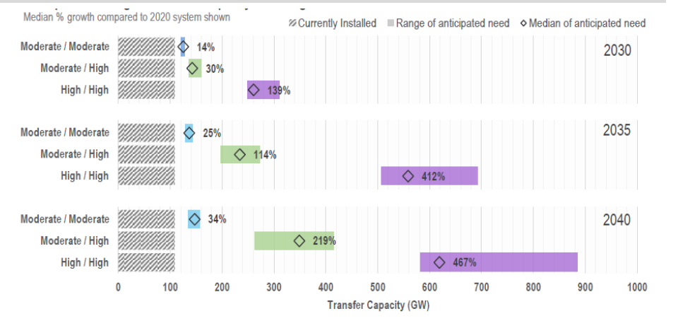
그림 9. 미국의 2035/2040년 지역간 송전용량의 요구치 전망
