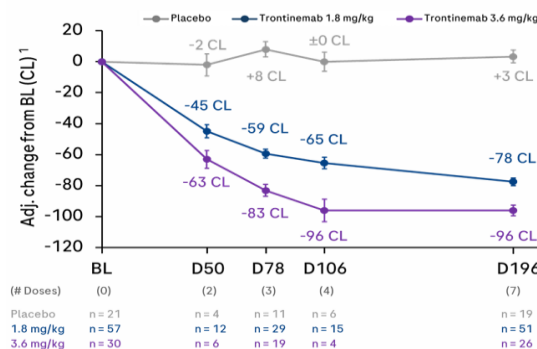
Trontinemab 투약 후 아밀로이드 감소 추이(28 주)
