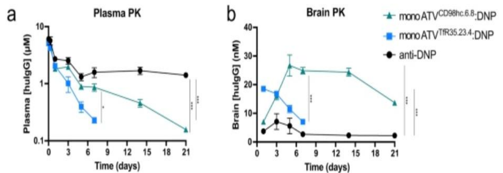
Plasma, Brain에서의 TfR, CD98hc ATV 비교
