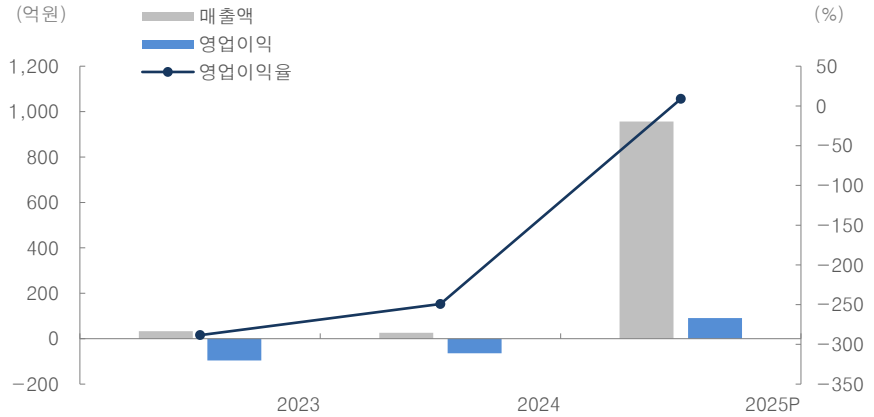
그림 1. 스피어 매출액 및 영업이익 추이 (연결기준)
